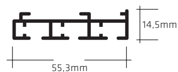
3 vias
