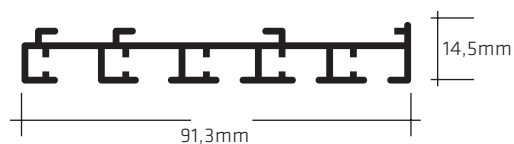
5 vias
